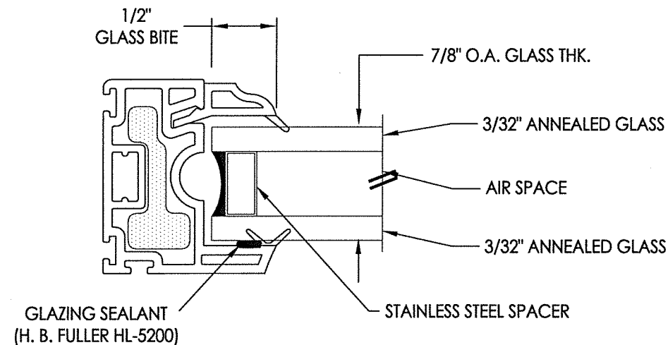
G2 GLAZING DETAIL
