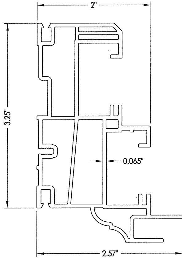
3 JAMB
